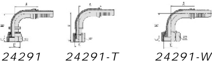
90° 美制 ORFS内螺纹平面 90° ORFS FEMALE FLAT SEAT ISO 12151-1- SAE J516
