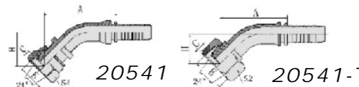
45° 公制内螺纹24° 锥带O形圈重系列 45° METRIC FEMALE 24° CONE O-RING H.T. ISO12151-2-DIN 3865
