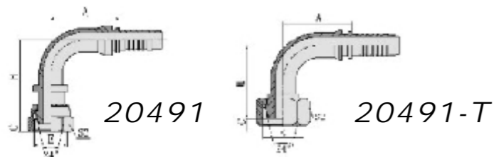
90° 公制内螺纹24° 锥带O形圈轻系列 90° METRIC FEMALE 24° CONE O-RING L.T. ISO12151-2-DIN 3865
