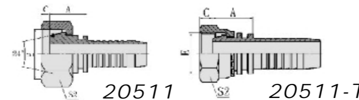
公制内螺纹24° 锥带O形圈轻系列 METRIC FEMALE 24° CONE O-RING H.T. ISO12151-1-DIN 3865
