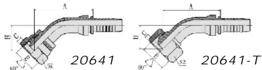
45° 公制内螺纹60° 外锥面 45° METRIC FEMALE 60° CONE
