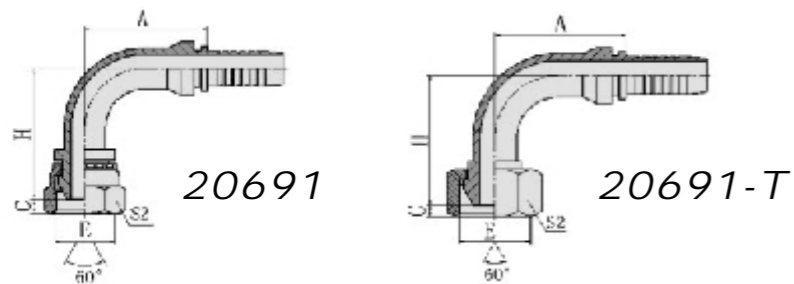
90° 公制内螺纹60° 外锥面 90° METRIC FEMALE 60° CONE
