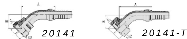
45° 公制内螺纹球面 45° METRIC FEMALE MULTISEAL
