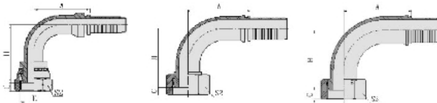
90° 英管内螺纹球面 90° BSP FEMALE MULTISEAL
