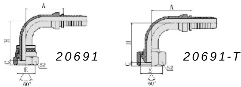
90° 公制内螺纹60° 外锥面 90° METRIC FEMALE 60° CONE
