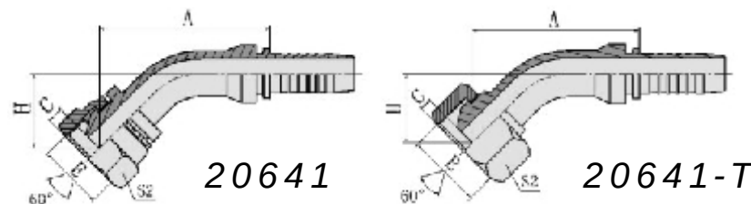
45° 公制内螺纹60° 外锥面 45° METRIC FEMALE 60° CONE
