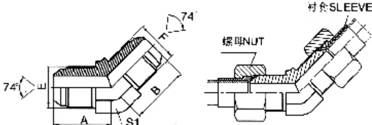
45 ° 弯美制JIC外螺纹74 ° 外锥 45 ° ELBOW JIC MALE 74 ° CONE
