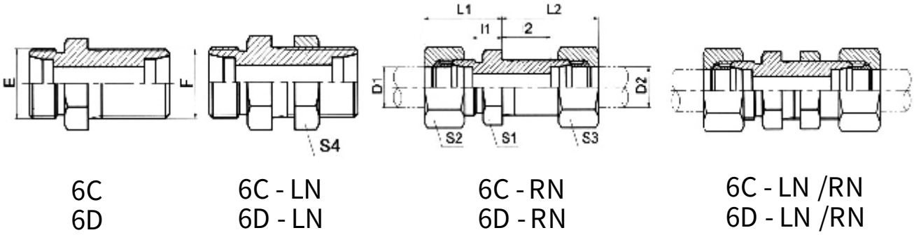
直通过板接头 STRAUGHT BULKHEAD FITTINGS
