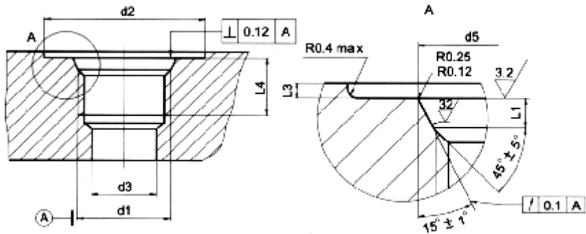
BS 5380 油口 Port
