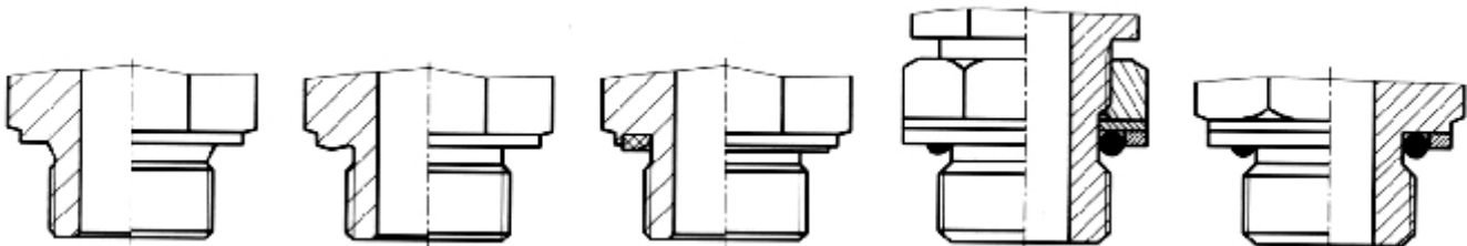
DIN 3852 A 型柱端 DIN 3852 Type A
