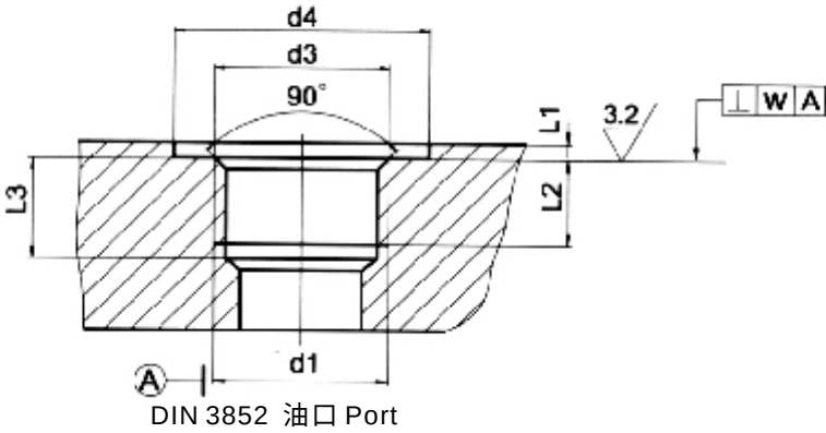
DIN 3852 油口 Port
