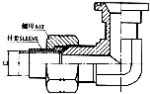
90° 弯美制JIC外落在74° 外锥 / 轻系列法兰ISO 6162-1 90° ELBOW JIC MALE 74° CONE / L-SERIES FLANGE ISO 6162-1
