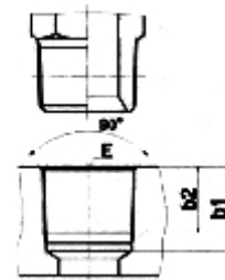
锥管螺纹油口 Taper Thread Port
