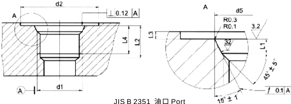
JIS B 2351 油口 Port 油口尺寸 Port Dimensions mm
