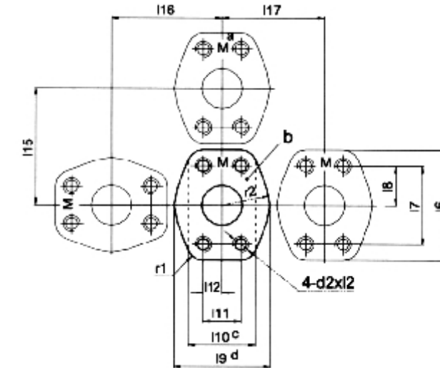
8 ISO6162 法兰油口 ISO 6162 Flange Port
