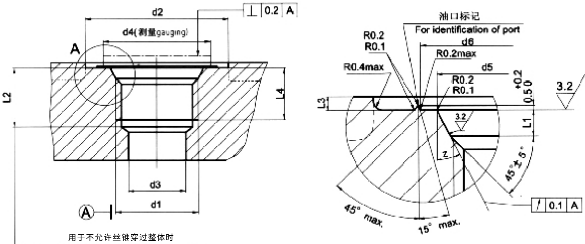
ISO 6149-1 油 口 Port
